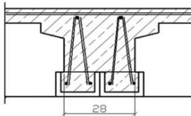
Doppelträger
