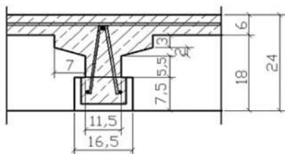
Einzelträger
