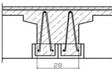
Doppelträger
