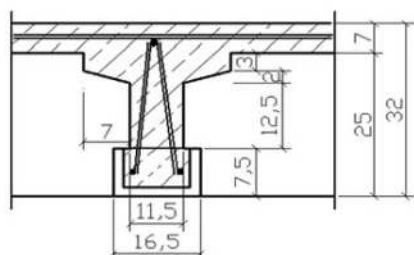
Einzelträger
