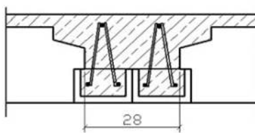
Doppelträger
