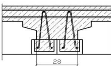
Doppelträger
