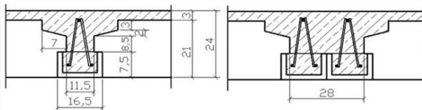
Einzelträger
