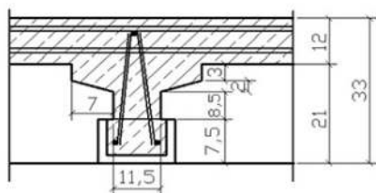
Einzelträger
