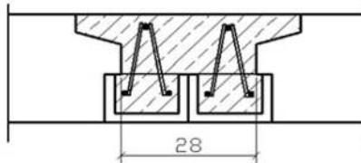
Doppelträger
