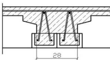
Doppelträger
