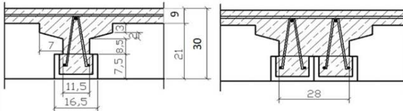
Einzelträger
