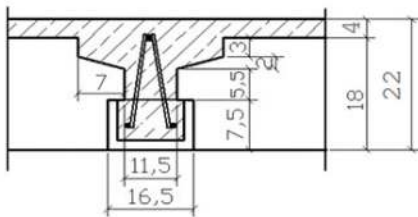
Einzelträger
