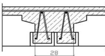
Doppelträger
