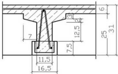
Einzelträger
