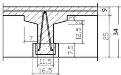
Einzelträger
