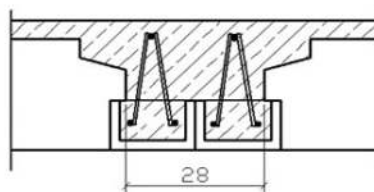
Doppelträger
