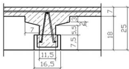
Einzelträger
