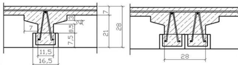
Einzelträger
