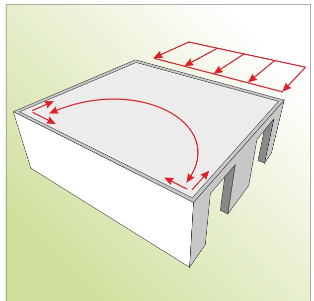
Scheibenwirkung der Decke: Die Ziegel-Einhängedecke wirkt als Druckbogen. Der umlaufende Ringanker leitet als Zugband die Horizontalkräfte in die Wandscheiben ab.
