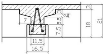
Einzelträger
